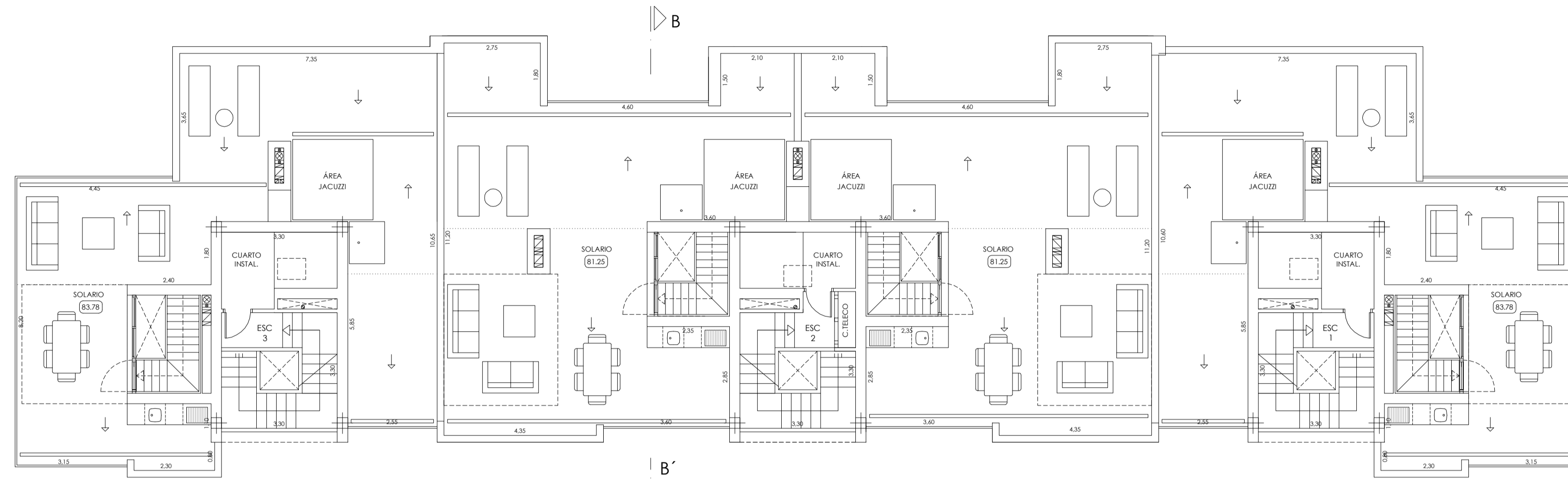
BLOQUE III. PLANTA CUBIERTA
