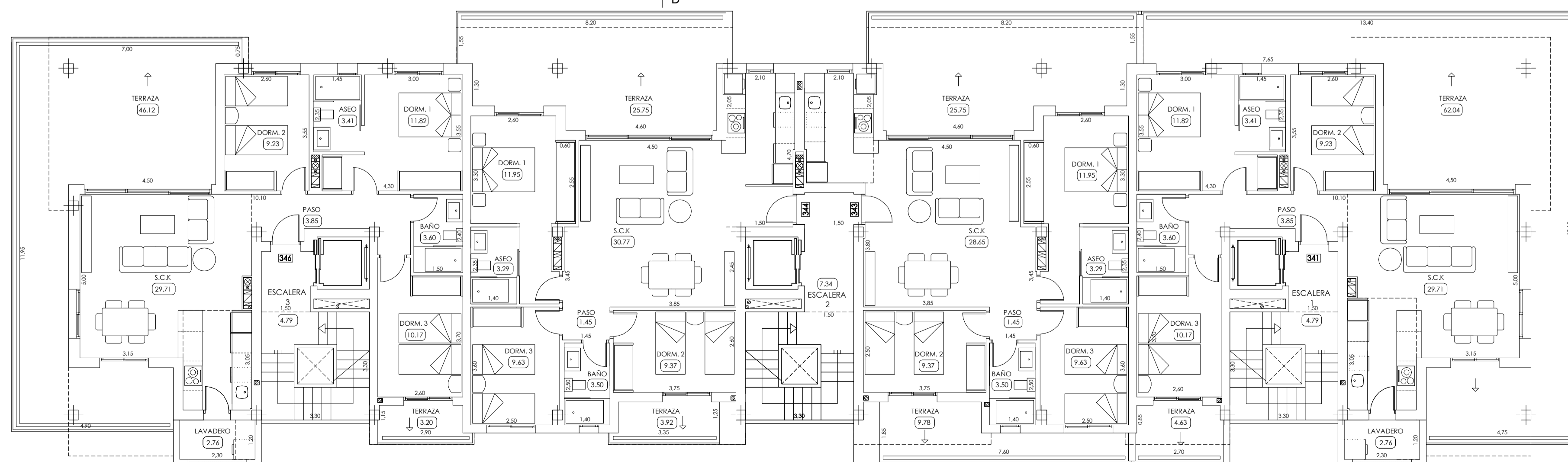
BLOQUE III. PLANTA 4
