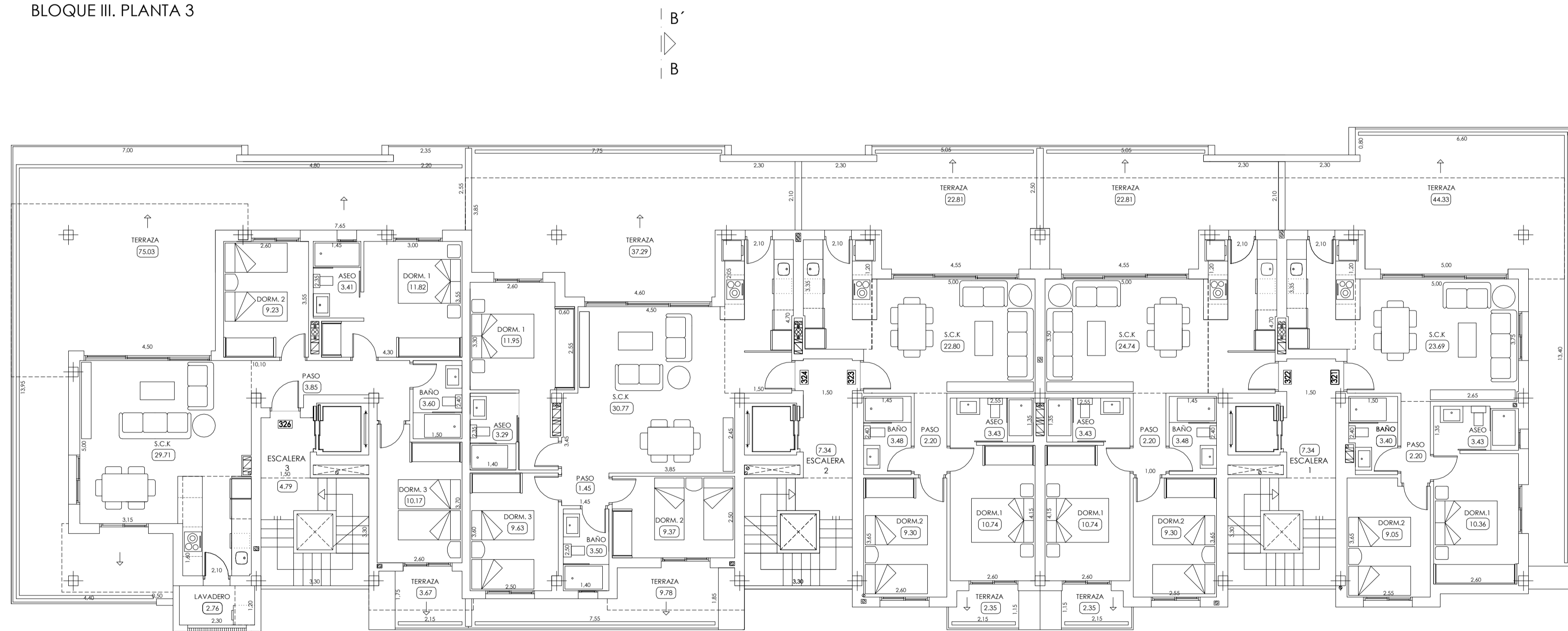
BLOQUE III. PLANTA 2
