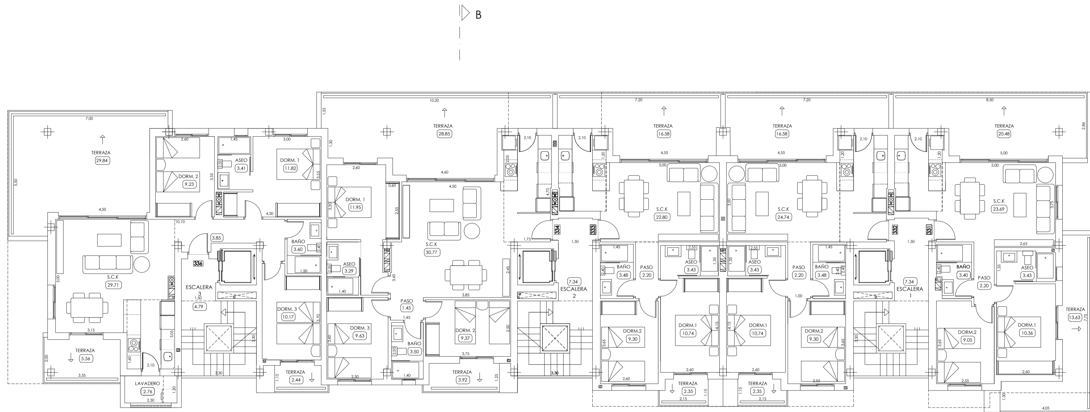
BLOQUE III. PLANTA 3
