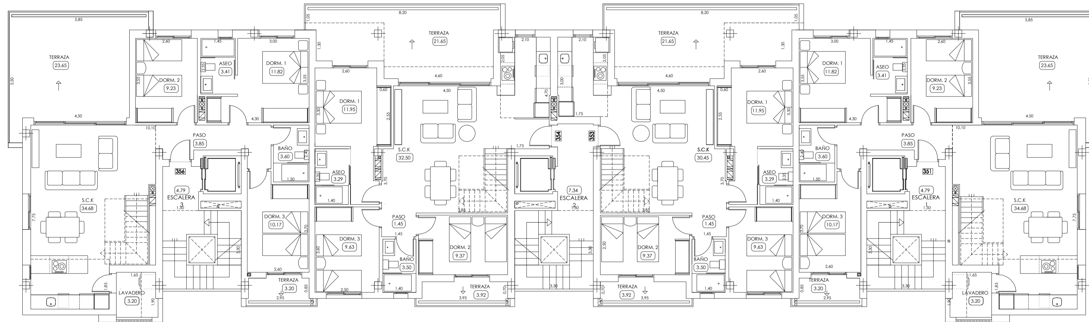
BLOQUE III. PLANTA 5
